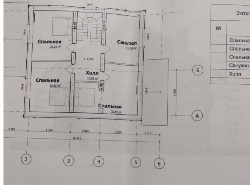
План второго этажа на отм.3,000 М (1:100)
