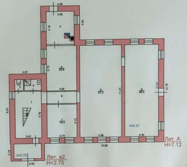
1 Этаж
