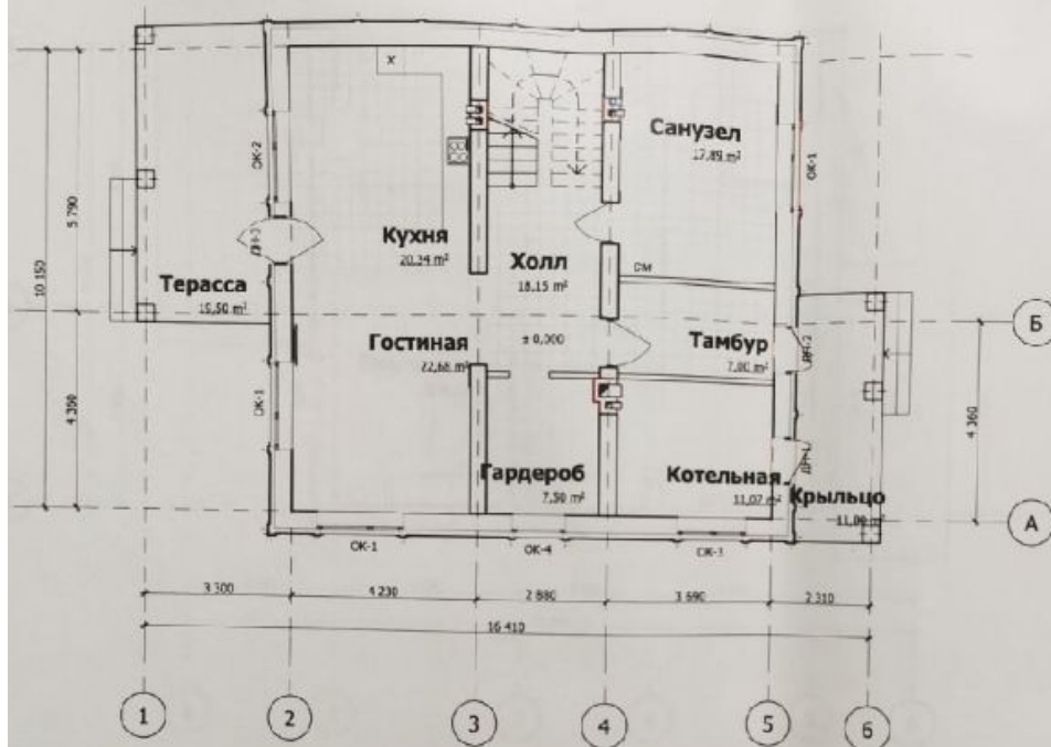
План первого этажа на отм.0,000 м (1:100)
