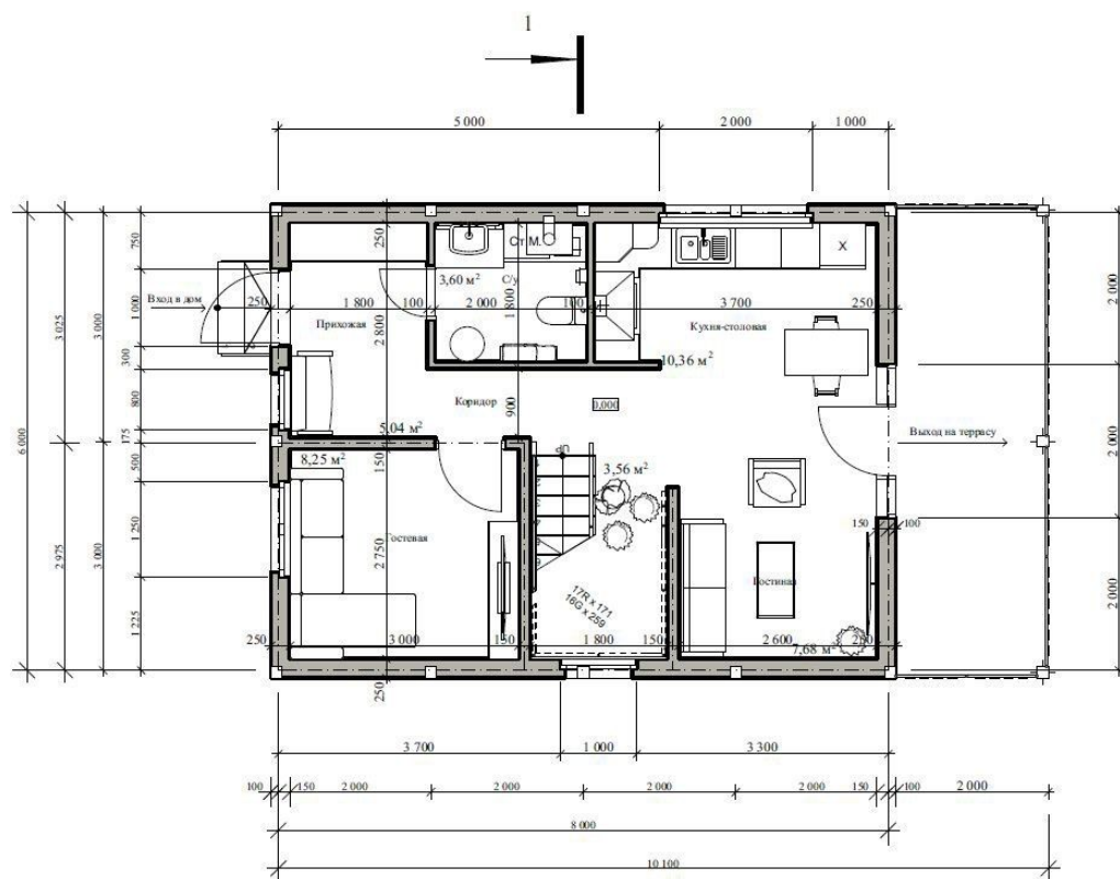
План 1-го этажа М 1:50
