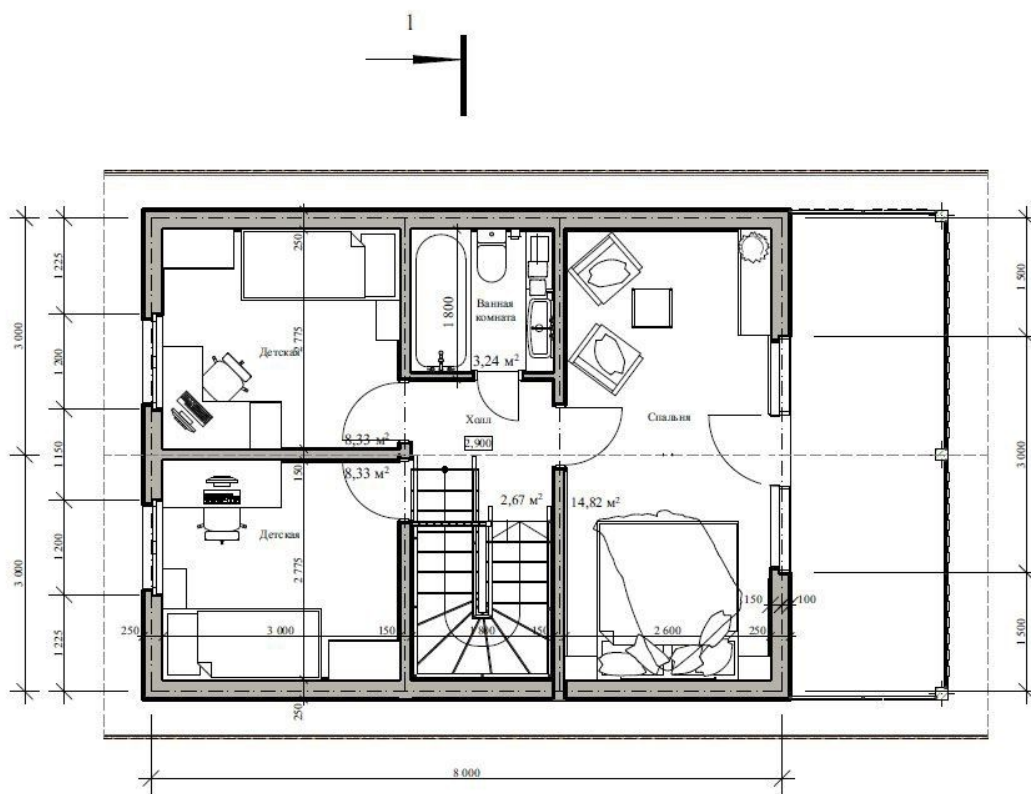
План 2-го этажа М 1:50
